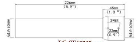
EC-SE45200mm
